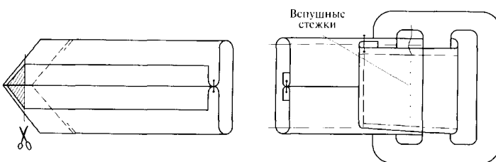
Рисунок 9 Обработка пояса с пряжкой
